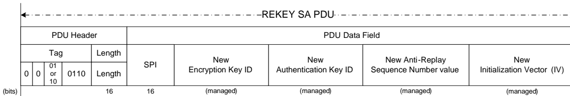
Figure 5-14: Rekey SA PDU
