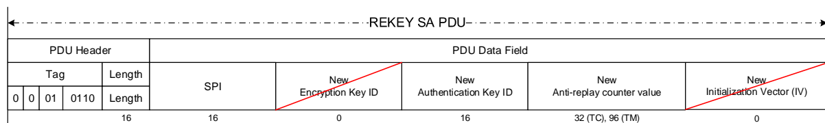
Figure D-8: Rekey SA PDU
